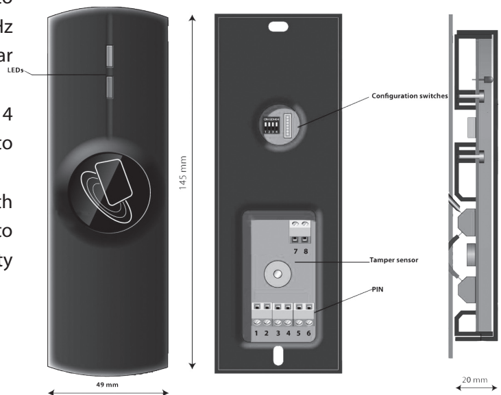
PIN Assignements
